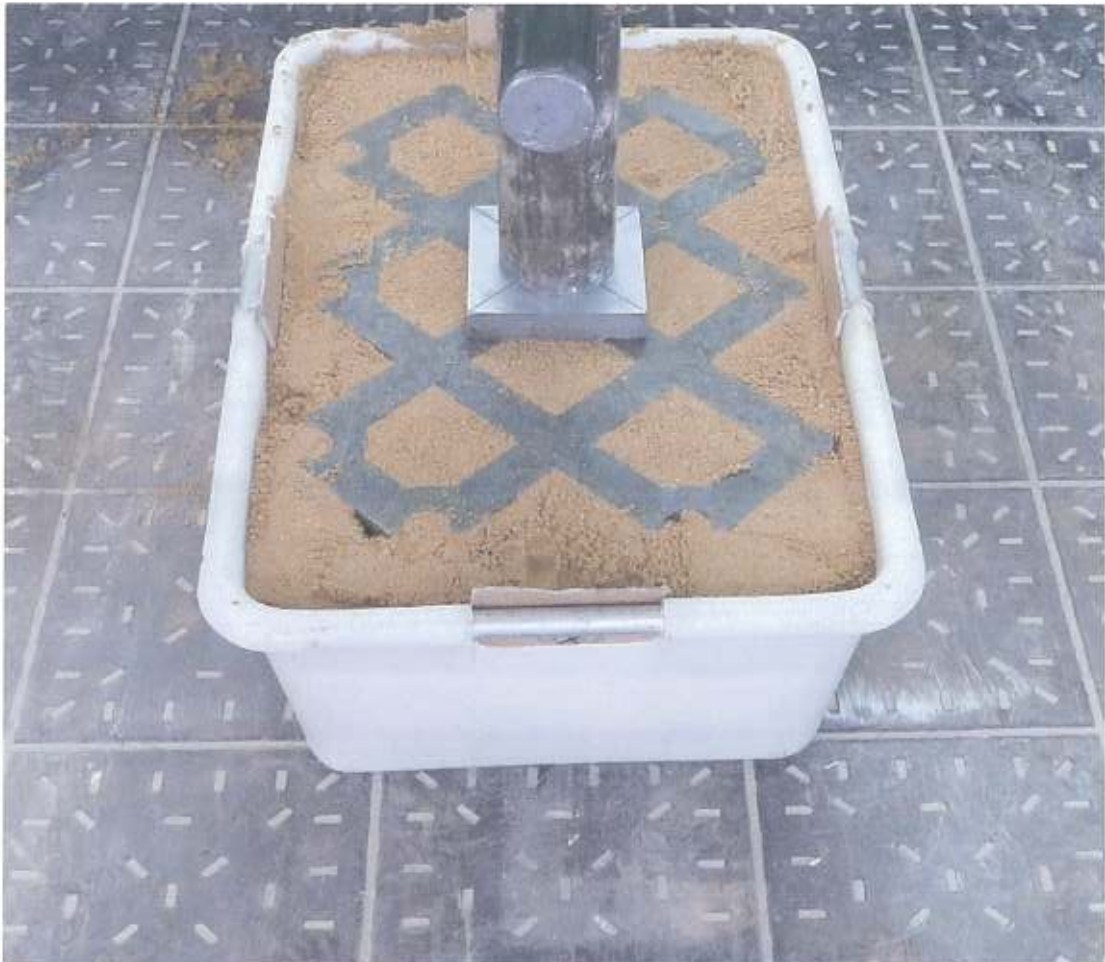
Abbildung 1: Prüfanordnung eines Kunststoffrasengittersteines auf künstlich hergestelltem Baugrund
