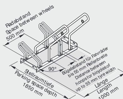
Modell 2502 XBF Model 2502 XBF
