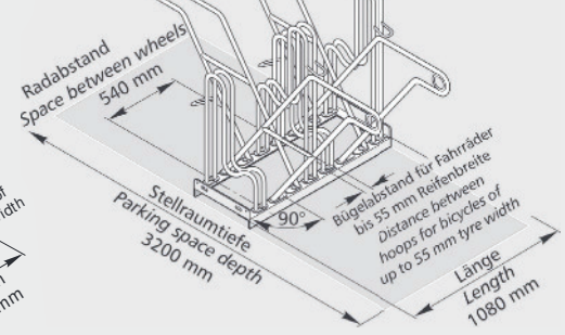
Modell 4614 XBF Model 4614 XBF
