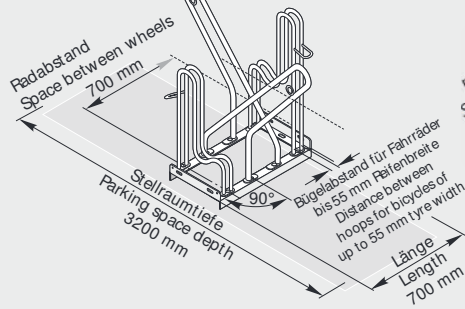
Modell 4602 XBF Model 4602 XBF
