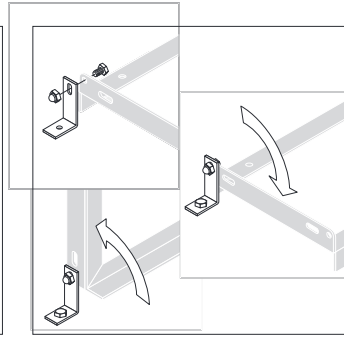
Optional Bodenmontage-Winkel, verzinkt (2er-Set). 4600 XBF: im Lieferumfang enthalten. Optional galvanised floor- mounting bracket (set of 2). 4500 XBF: ind. in scope of delivery
